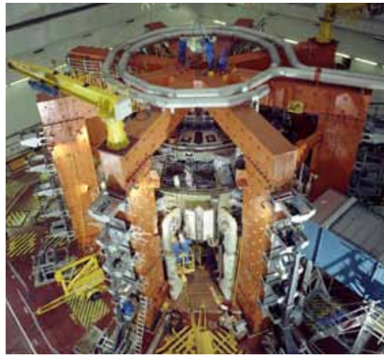
Buitenkant van de Joint European Torus (JET) in het Verenigd Koninkrijk. © EFDA-JET
